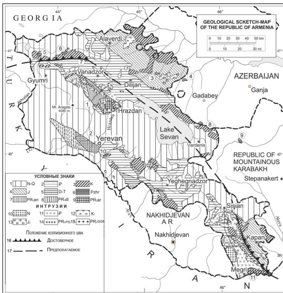
Рис. 1. Положение шва континентальной коллизии Перигондванского (Киммерийского) континента (Ю-З область) с южной периферией Евразийского континента (С-В область) в верхнемеловое время. Условные обозначения: отложения: 1 – неоген-четвертичные; 2 – палеогеновые; 3 – меловые; 4 – юрские; 5 – палеозойские (девон-пермь) и триасовые; метаморфические породы кристаллического фундамента: 6 – метаморфический палеозой герцинского фундамента евроазиатской окраины мезозоя; 7–9 – докембрийский кристаллический фундамент Перигондванской складчатой зоны Армении: 7 – верхний протерозой, Анкаванская серия; 8 – верхний протерозой, Далларская серия; 9 – средний протерозой, Арзаканская серия; интрузивные комплексы: 10 – неогеновые; 11 – палеогеновые; 12 – нижнемеловые; 13 – юрские; 14 – верхнепротерозойские трондьемиты; 15 – верхнепротерозойские гранито-гнейсы.
