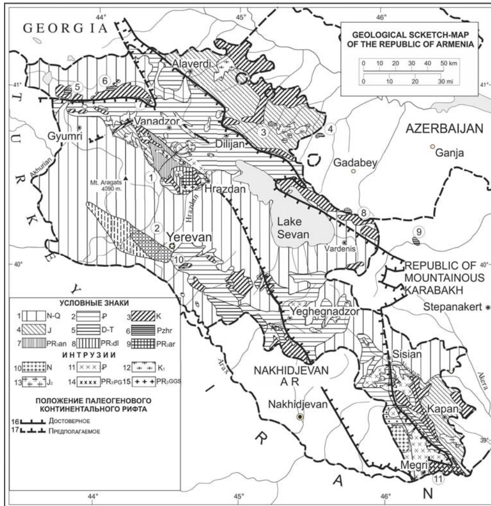
Рис. 2. Контуры Ширак-Севан-Мегринского палеогенового рифта на схематической геологической карте Армении.
