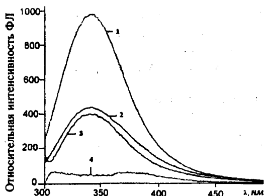
Рис. 1. Спектры ФЛ раствора аргиназы (рН 6, концентрация -4 \cdot 10^{-7}\text{М} ) при \lambda_{\text{возб}}=280\text{нм} (1), 257\text{нм} (2), 297\text{нм} (3); разностный спектр ФЛ (4).
