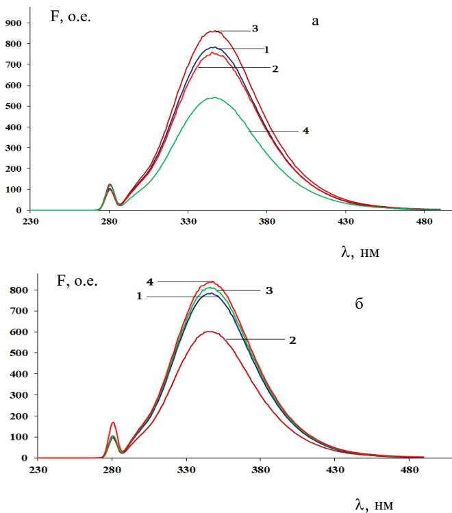
Рис. 2. Спектры флуоресценции необлученных (кривая 1) и облученных (кривые 2-4) образцов альбумина. Образцы альбумина облучены частотой 41,8 ГГц (а) и 51,8 ГГц (б). Кривые 2 соответствуют спектрам флуоресценции, которые получены непосредственно после облучения, кривые 3 – через 24 часов после облучения, кривые 4 – через 48 часов после облучения.
